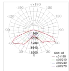
80°*150°PC lens
