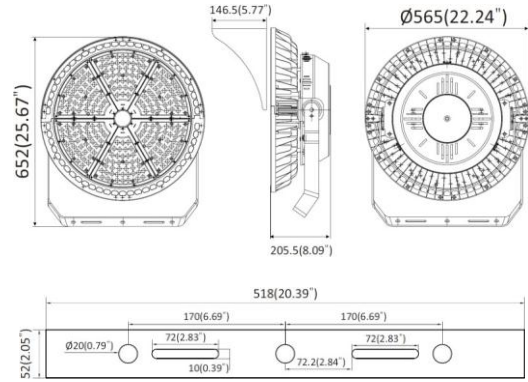
MAS-FL-UF500J / MAS-FL-UF600J / MAS-FL-UF700J
