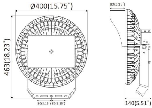
MAS-FL-UF200J / MAS-FL-UF300J / MAS-FL-UF400J
